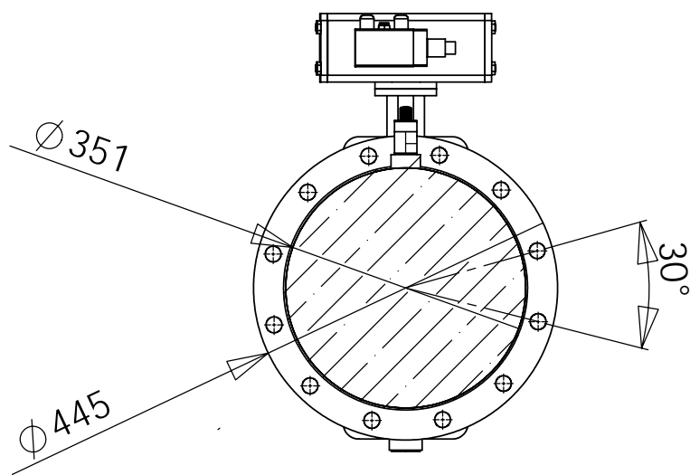
COUPE A-A ECHELLE 1 : 10
