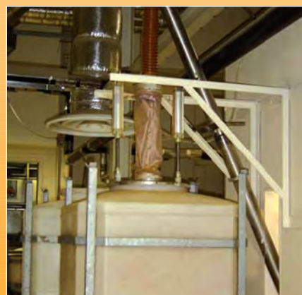
Station de remplissage confinée
