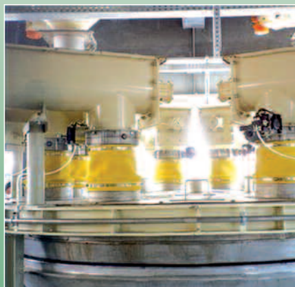
Vanne en bout de vis pour optimisation de dosage
