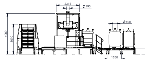
➤ Dosage et pesage : automatisation et ergonomie du poste de travail
